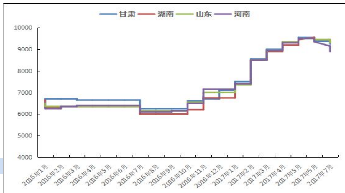
图 2、2016 年-2017 年 7 月主流地区氟化铝月度价格统计
