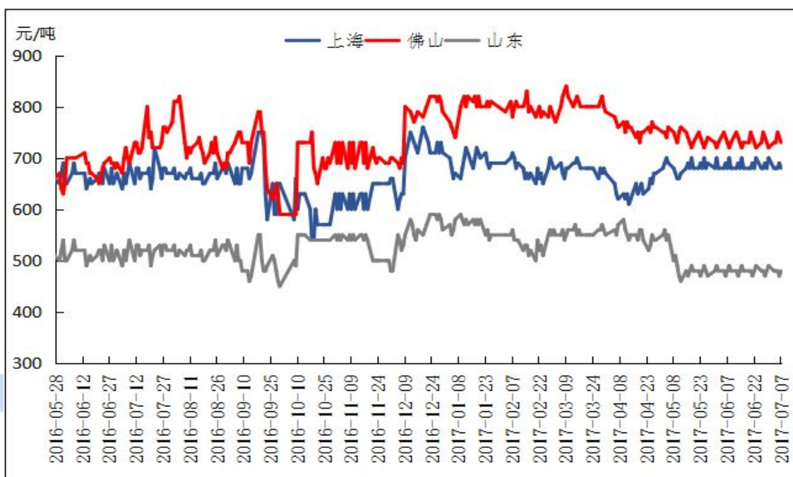
图6、全国主流地区 A356.2 铝合金锭加工费走势图 规格：国标
