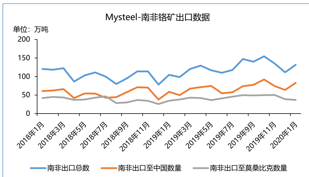
图二 Mysteel 南非铬矿出口数据
