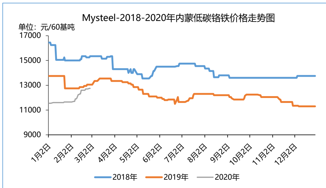
图七 Mysteel 内蒙低碳铬铁价格走势
