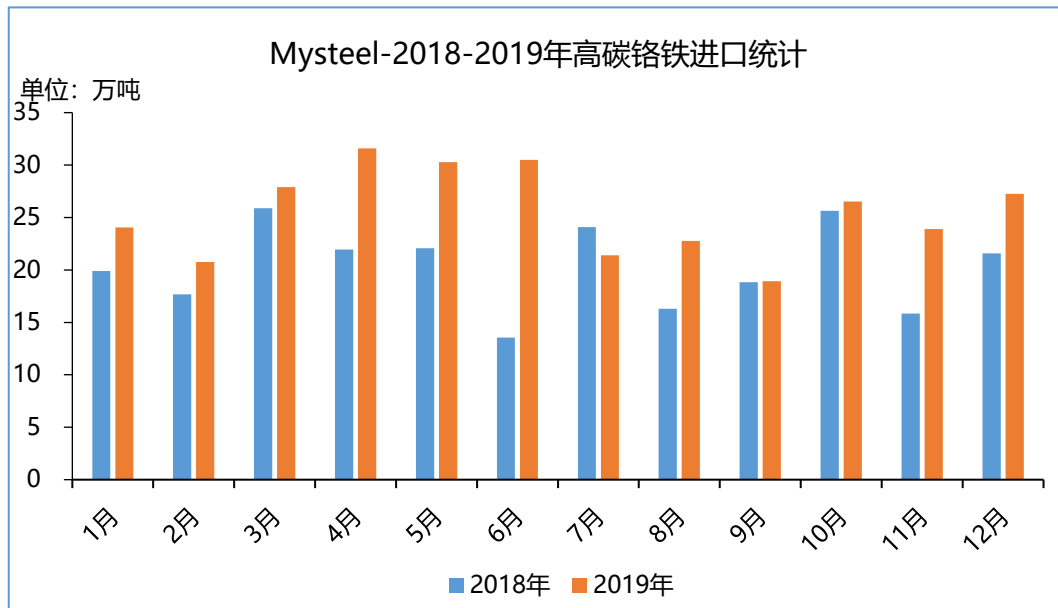
图九 Mysteel2018-2019 年高碳铬铁进口统计
