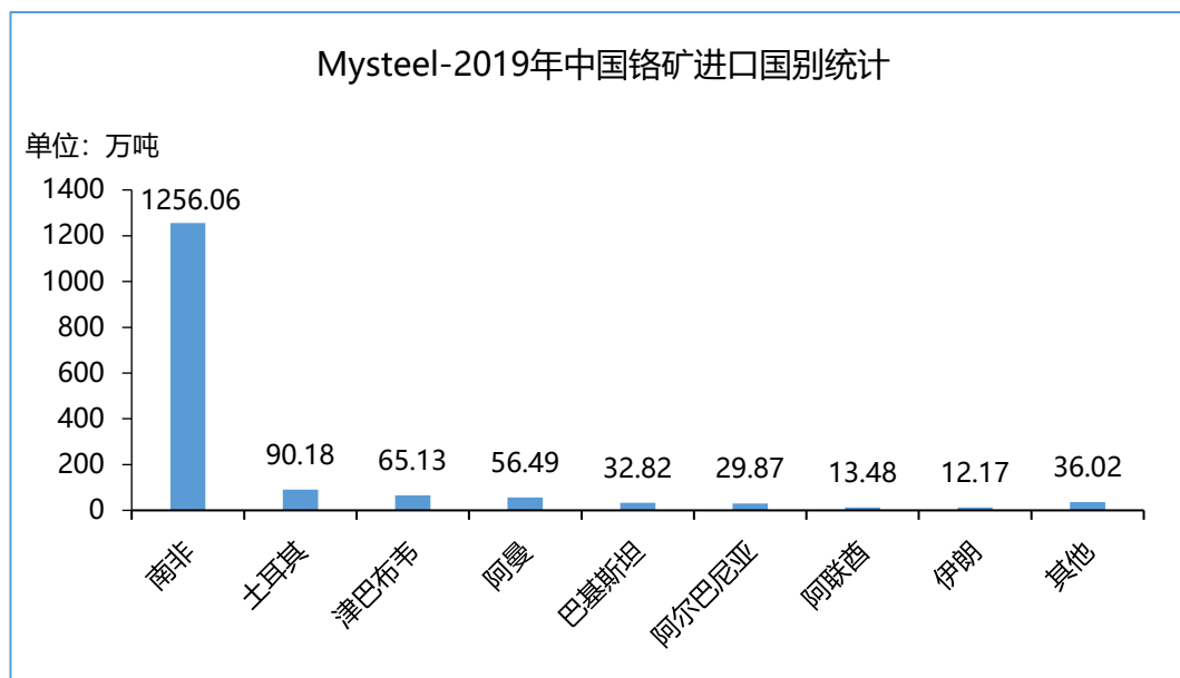
图三 Mysteel2019年中国铬矿进口国别统计
