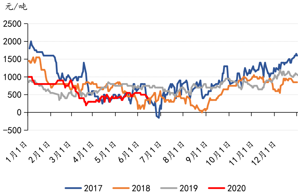
Mysteel: 304冷轧-热轧价差
