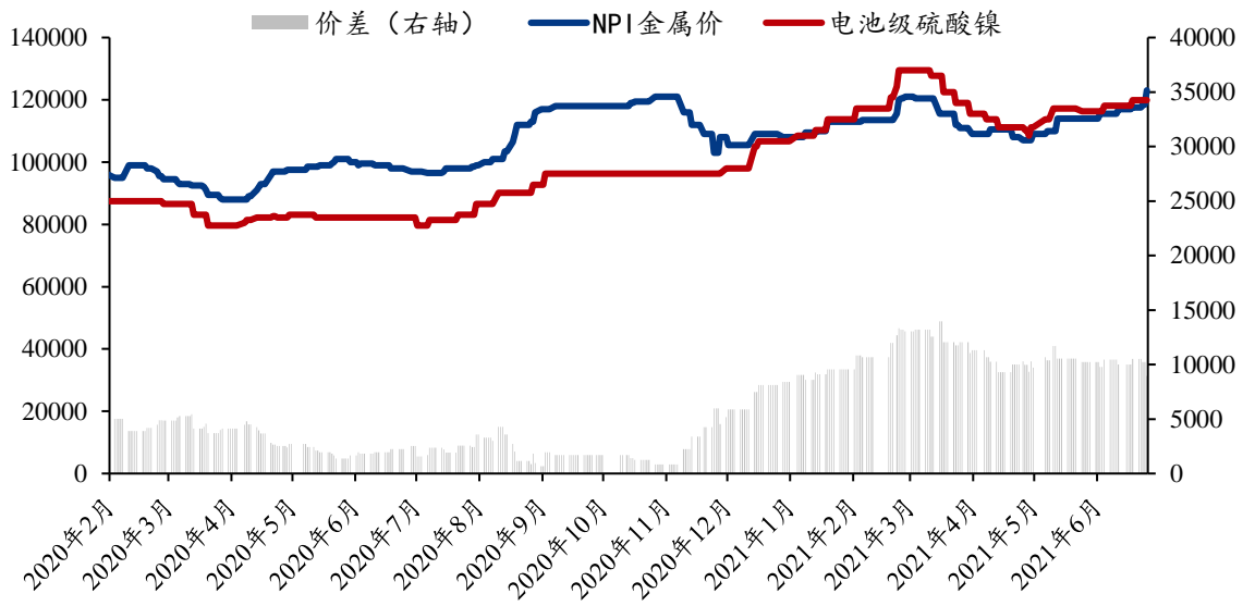
Mysteel-硫酸镍与镍铁价差(元/吨)
