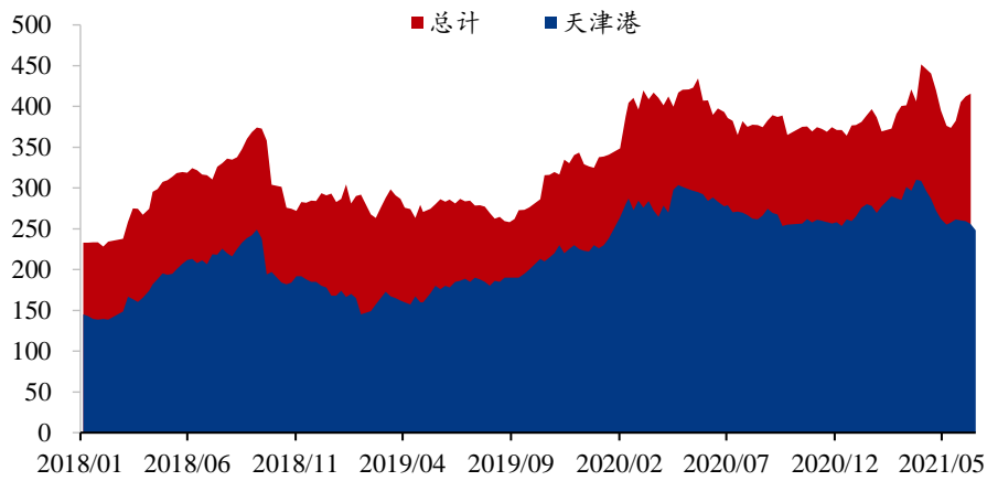
Mysteel-铬矿港口库存变化趋势(万吨)
