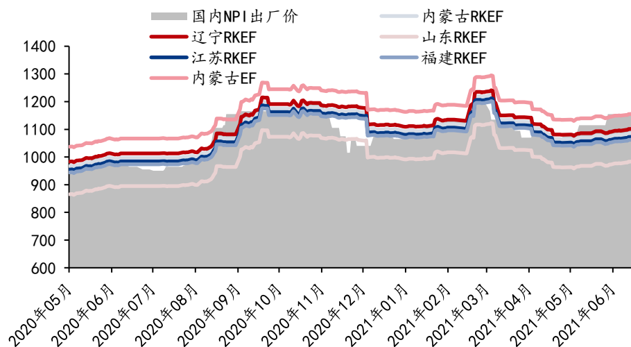
Mysteel 国内镍铁即期成本 (元/镍)
