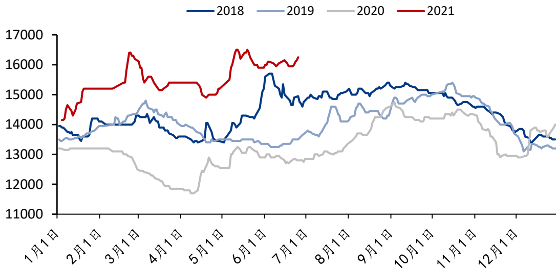
Mysteel 无锡市场东方特钢304热轧价格走势（元/吨）
