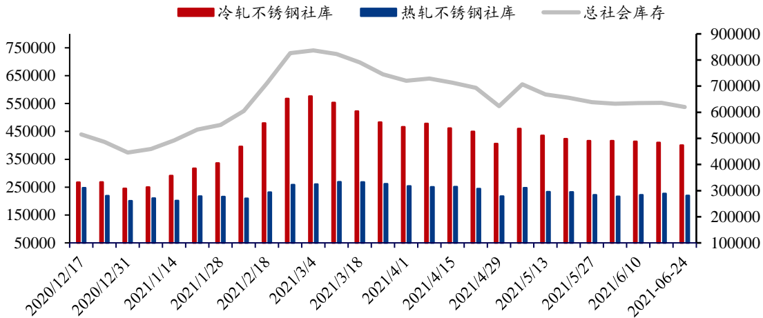
Mysteel新口径不锈钢社库合计（单位：吨）
