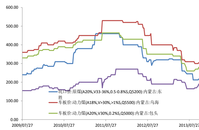
图表 18 内蒙古动力煤坑口价
