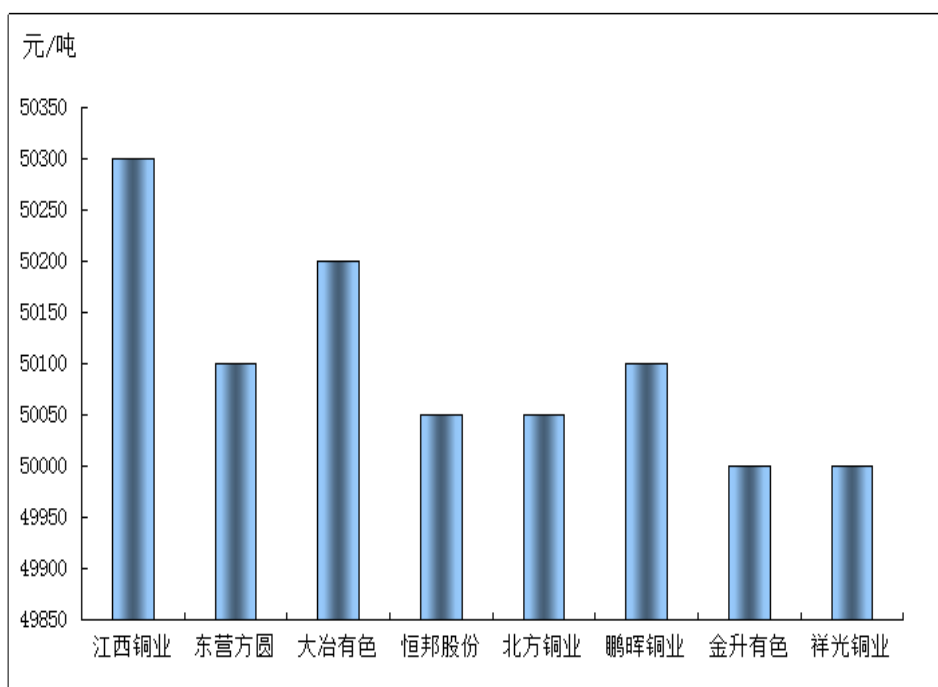
图一 4日铜企出厂价格统计
