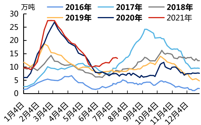
图12：6063铝棒库存变化走势图
