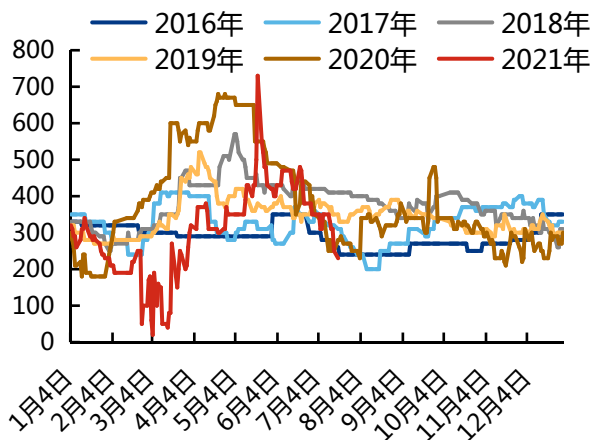
图11：无锡地区 6063 铝棒加工费走势图
