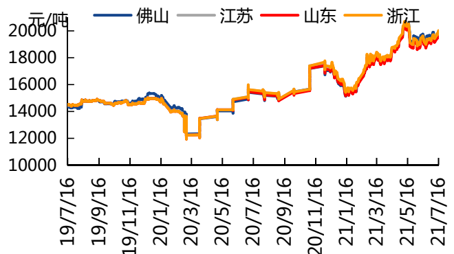
图16：中国主流地区A356.2价格走势图
