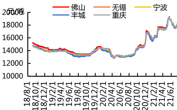
图15：中国主流地区ADC12格走势图
